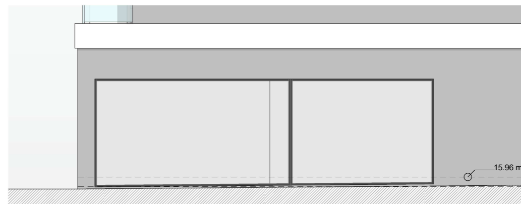
Alzado Sur 1:100 (A3)
